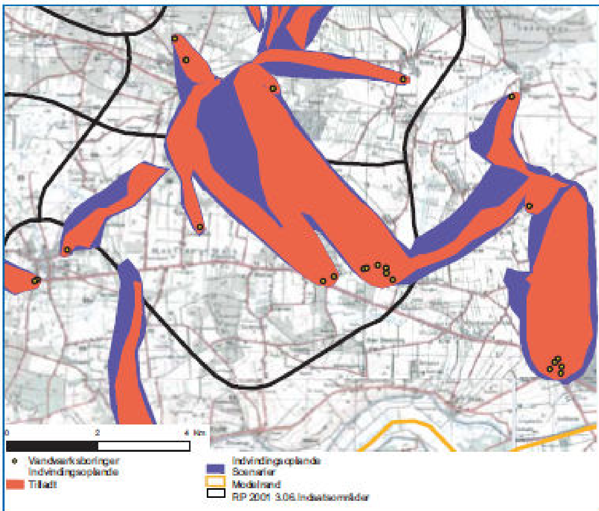
Figur 5.6 .Indvindingsoplande beregnet med den hydrologiske model i relation til indsatsområde Kastbjerg.
