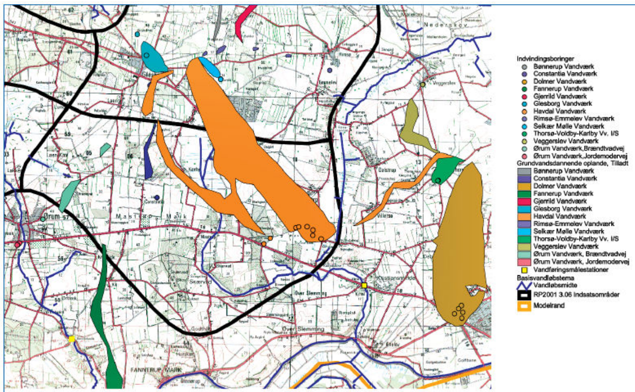
Figur 5.4. Grundvandsdannende oplande beregnet ved basis scenariet i relation til indsatsområde Kastbjerg.
